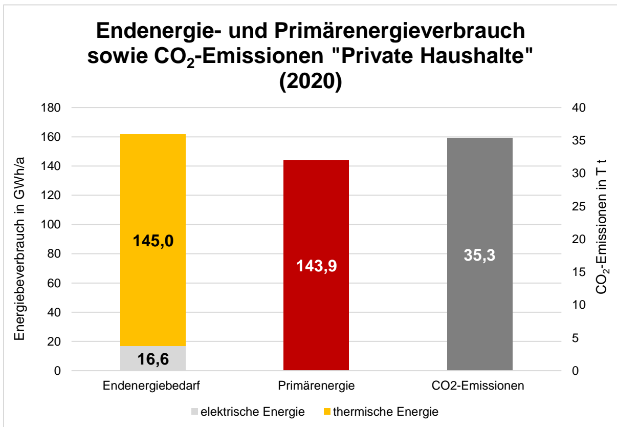
Abbildung 15: Endenergie- und Primärenergieverbrauch in GWh/ a sowie CO 2 -Emissionen in der Verbrauchergruppe „Private Haushalte“ in T t/ a 2020
