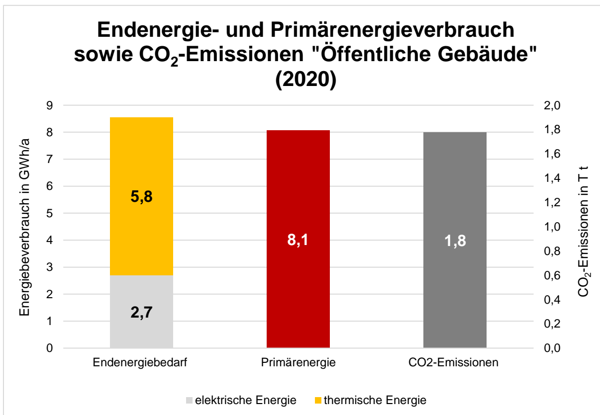
Abbildung 17: Endenergie- und Primärenergieverbrauch in GWh/ a sowie CO 2 -Emissionen in der Verbrauchergruppe „Öffentliche Gebäude“ in T t/ a 2020
