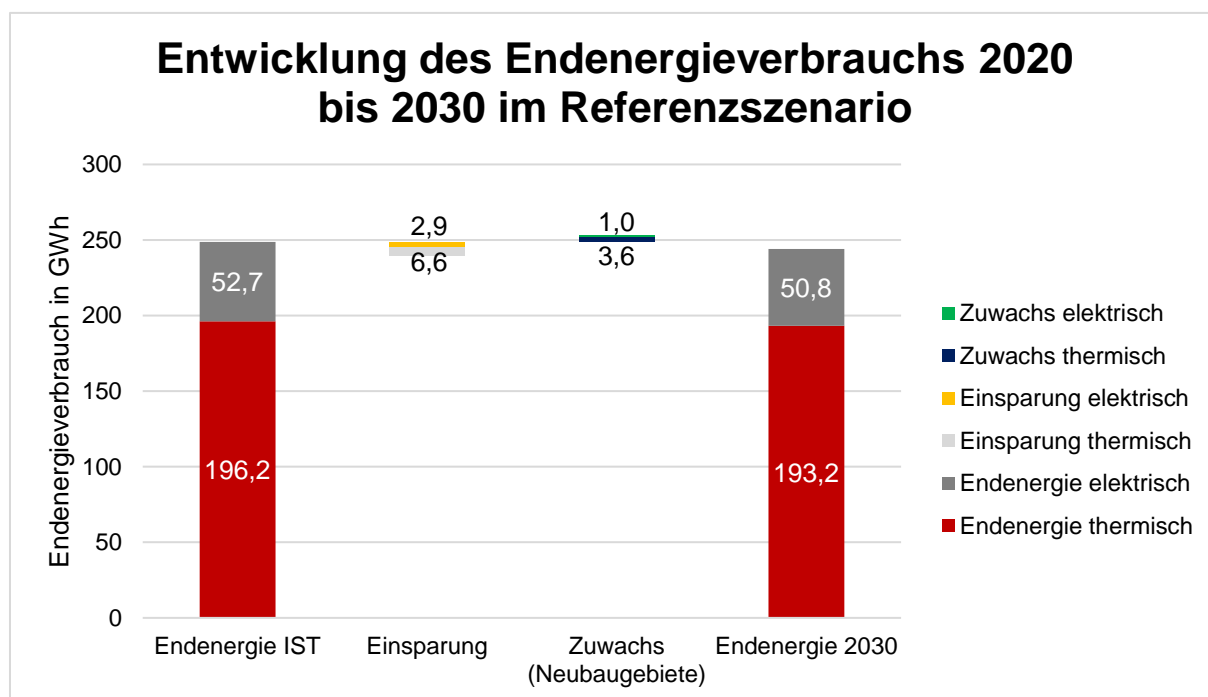
Abbildung 34: Potenzial Reduktion Endenergieverbrauch Referenzszenario
