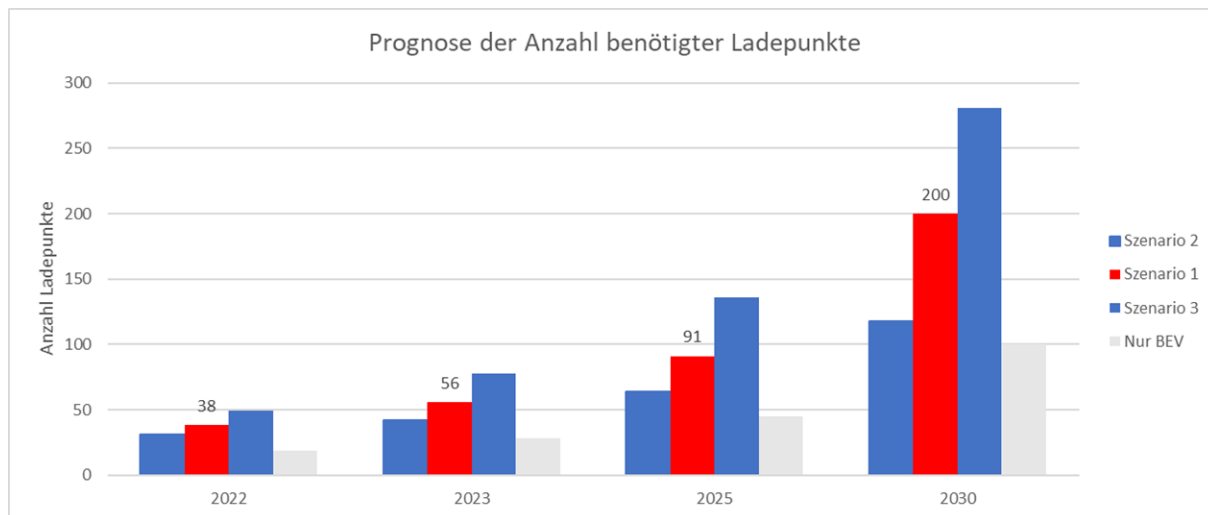
Abbildung 51: Prognose der benötigten Ladepunkte auf Basis des T-Wertes der EU-Kommission
