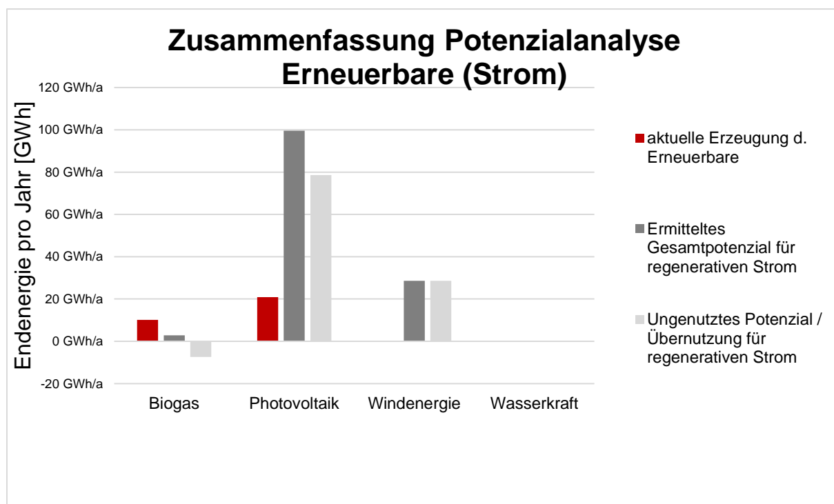
Abbildung 46: Zusammenfassung Potenzialanalyse Erneuerbare (Strom)
