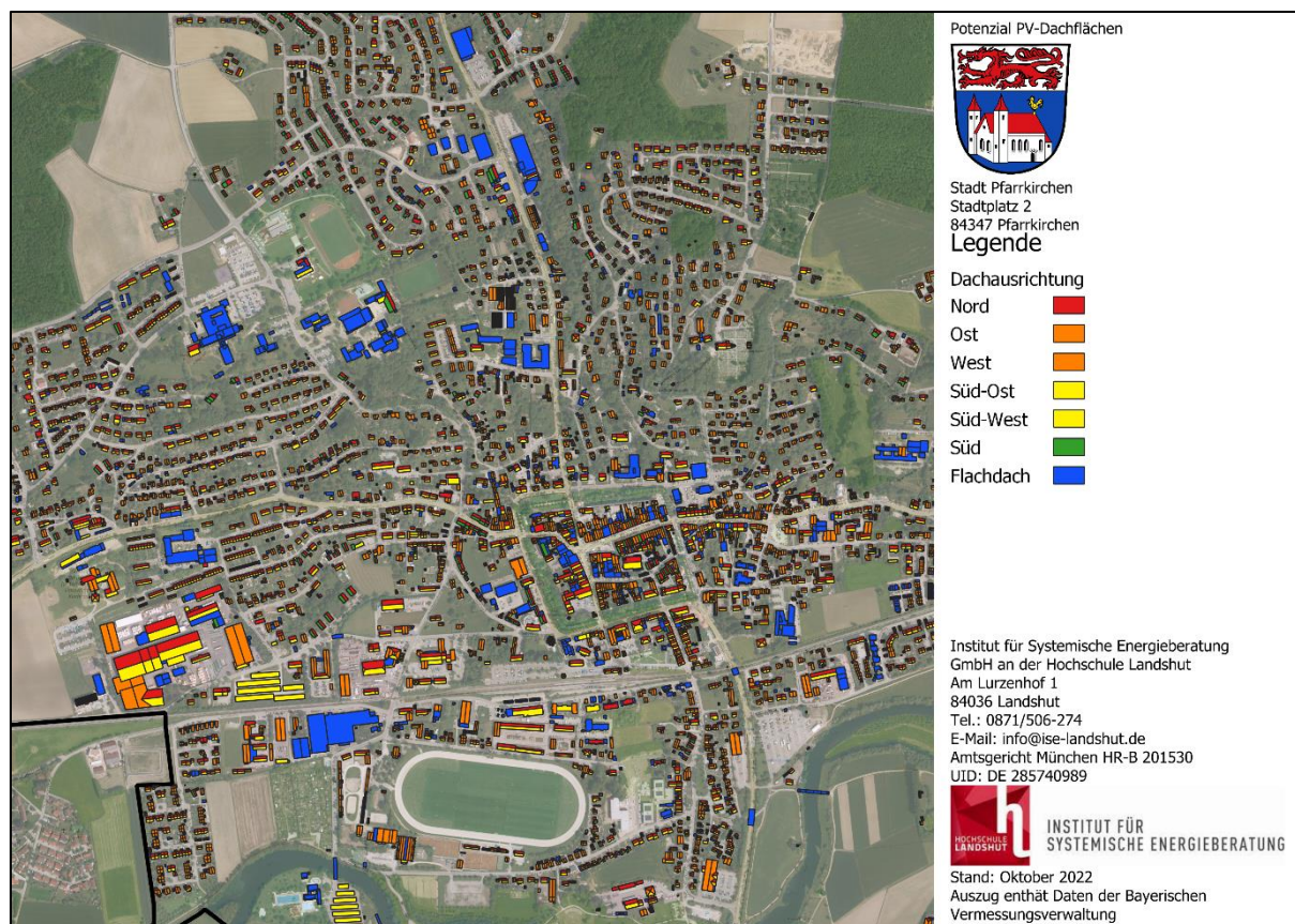
Abbildung 44: Solarpotenzial Dachflächen Pfarrkirchen
