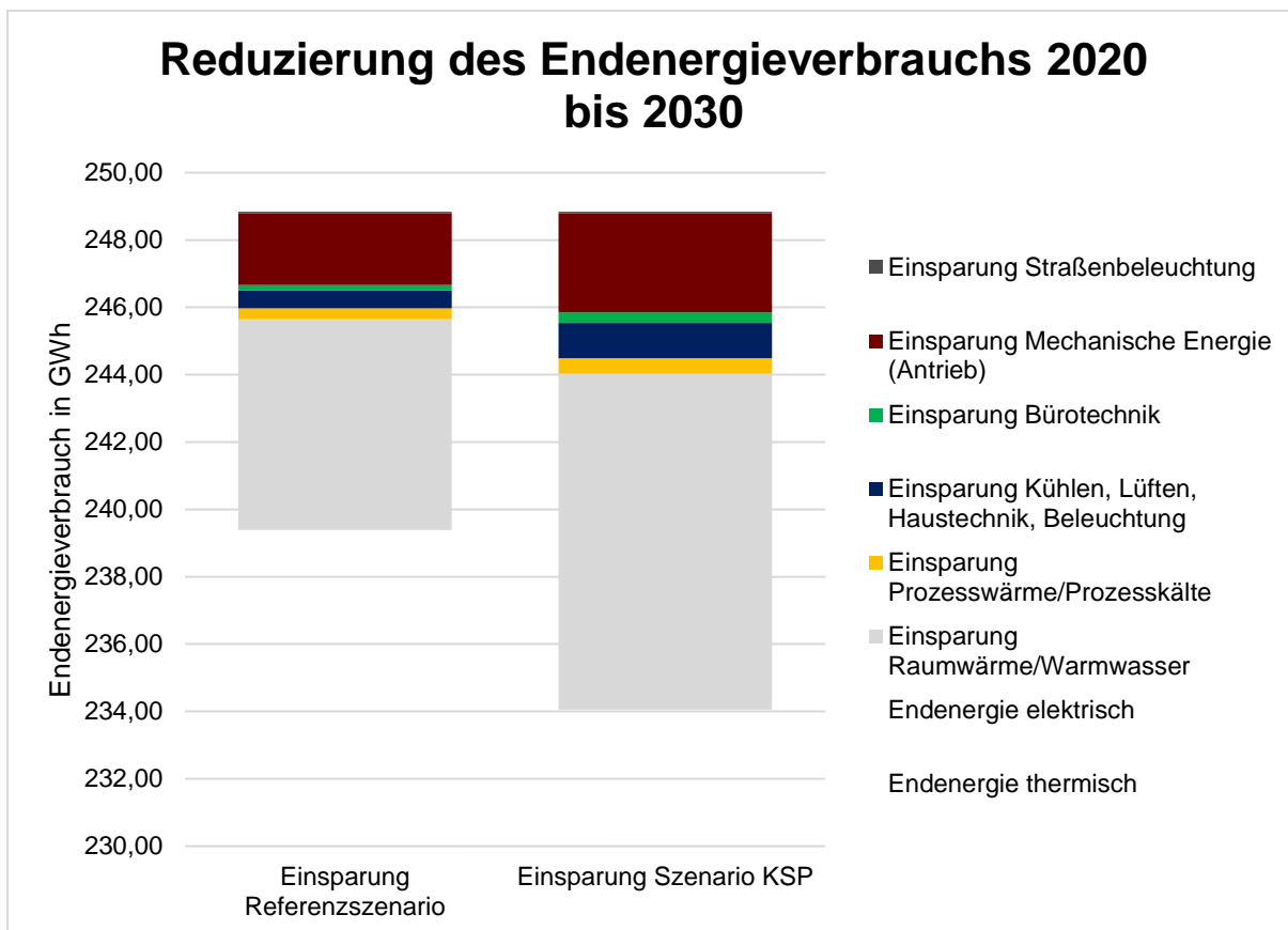
Abbildung 36: Reduktion des Endenergieverbrauchs nach Szenarien und Ansatzpunkten/ Verwendungszwecken
