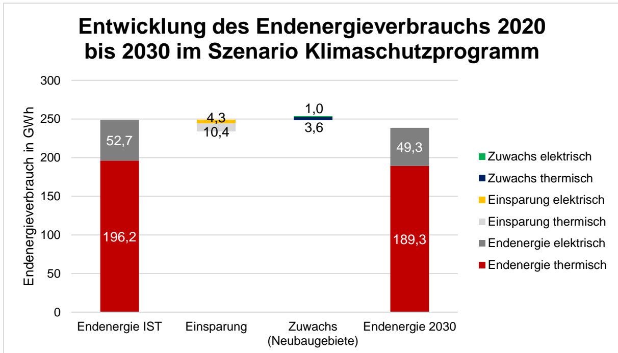
Abbildung 35: Potenziels Reduktion Endenergieverbrauch Klimaschutzprogramm
