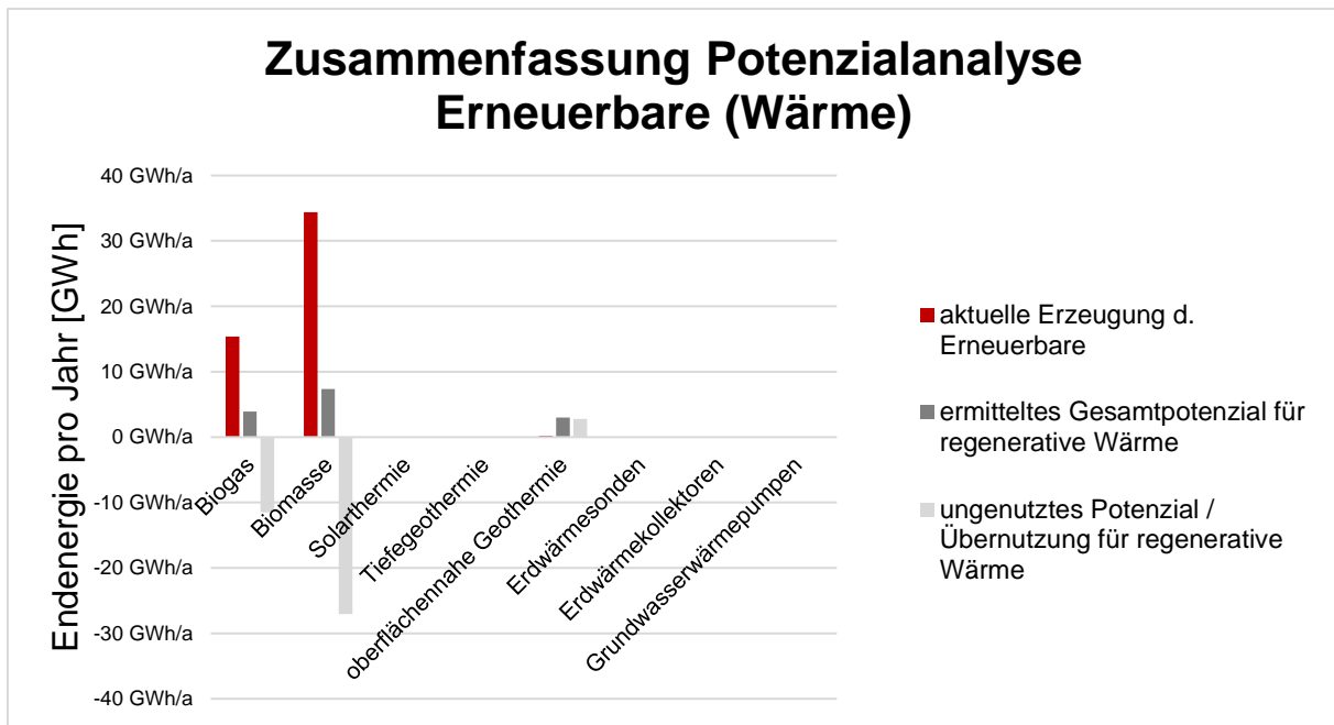
Abbildung 47: Zusammenfassung Potenzialanalyse Erneuerbare (Wärme)
