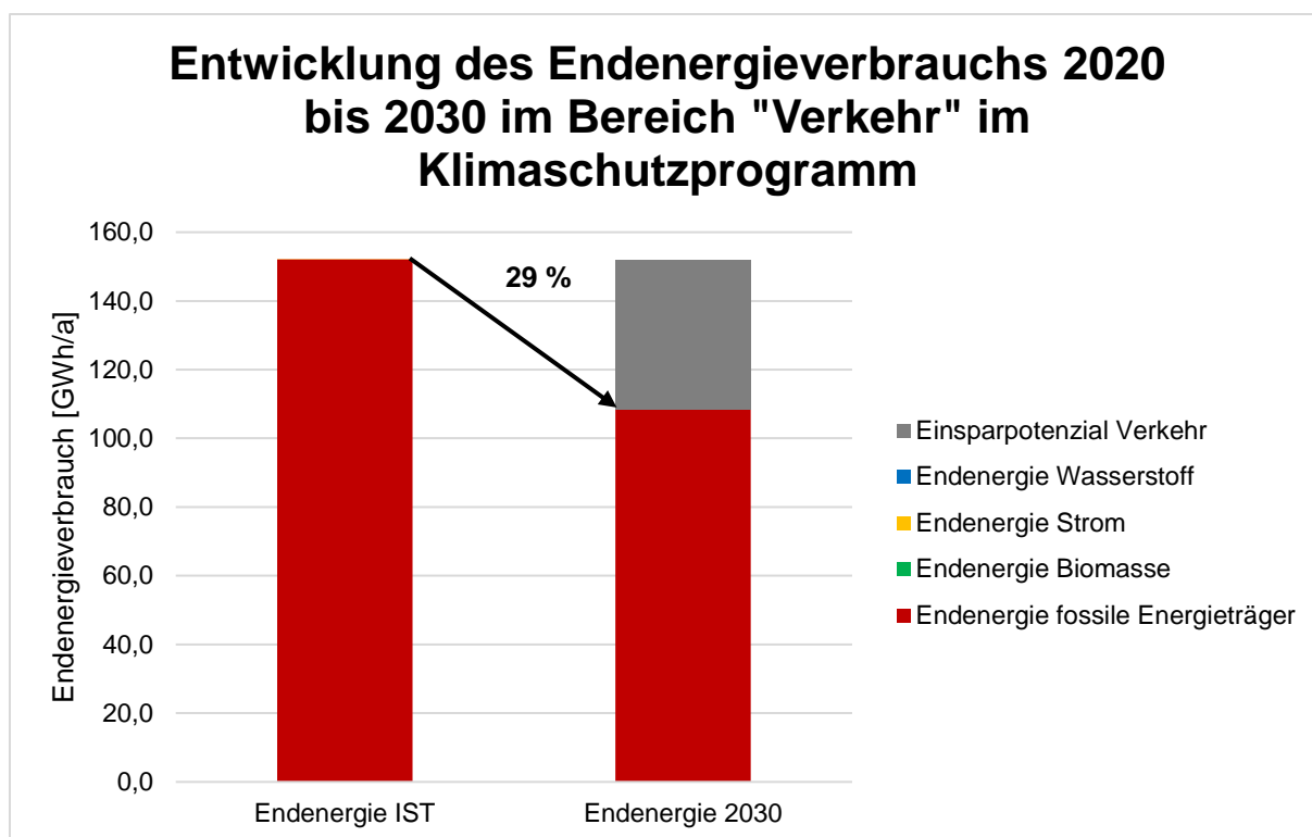
Abbildung 38: Potenzial Reduktion Endenergieverbrauch im Bereich "Verkehr" Klimaschutzprogramm
