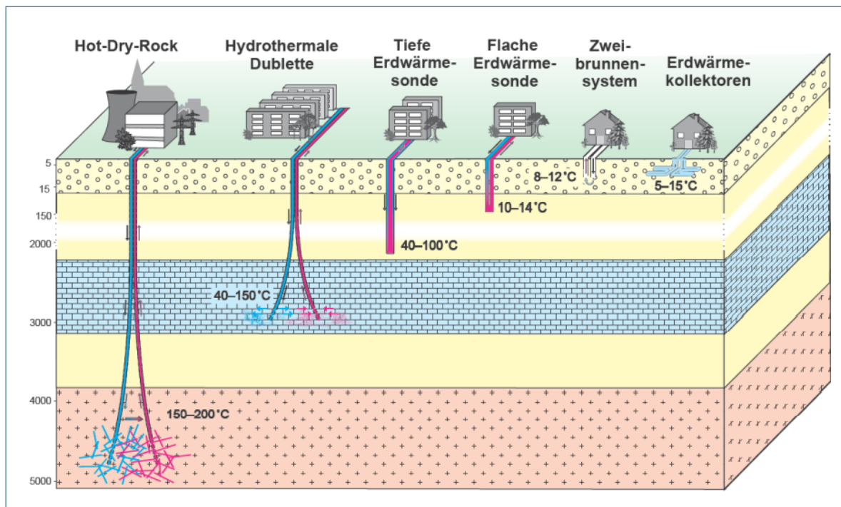
Abbildung 40: Nutzung der Erdwärme im Vergleich
