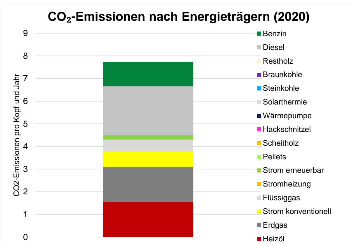
Abbildung 21: CO 2 -Emissionen nach Energieträgern in t/Kopf 2020 in Pfarrkirchen
